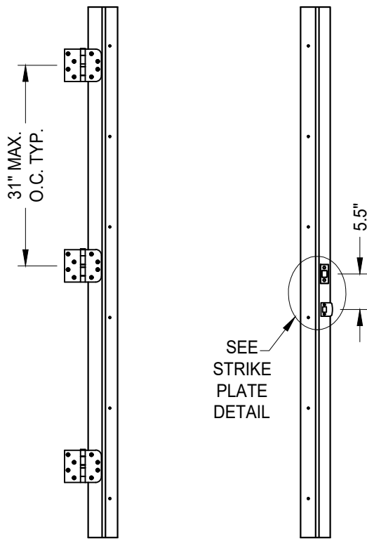
HINGE JAMB
